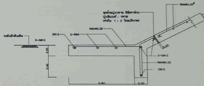
รายละเอียด 1 NOT TO SCALE
