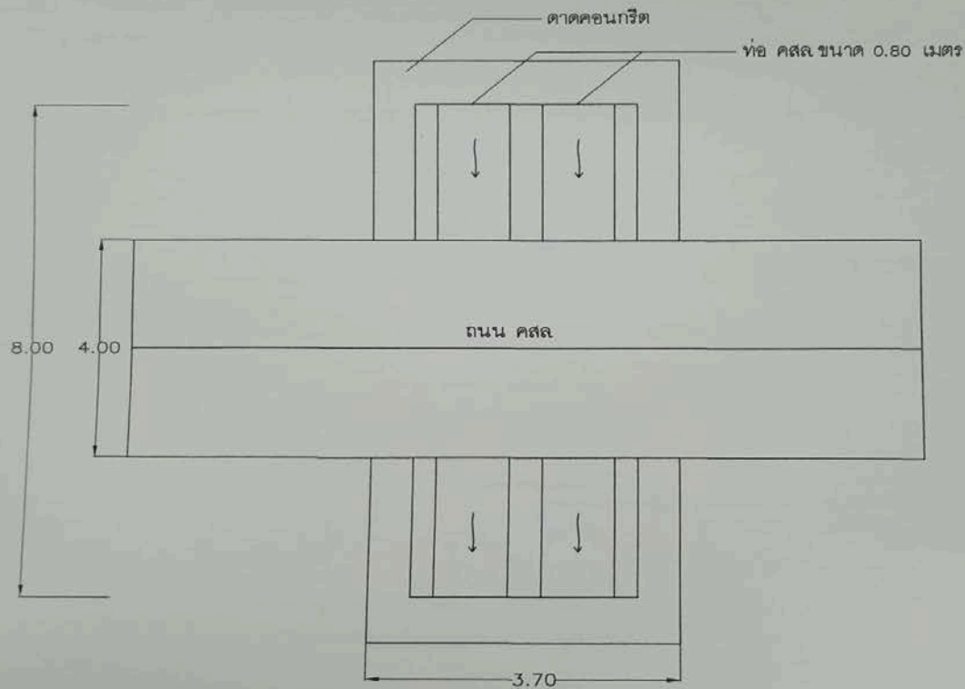
แบบแปลนท่อ NOT TO SCALE
