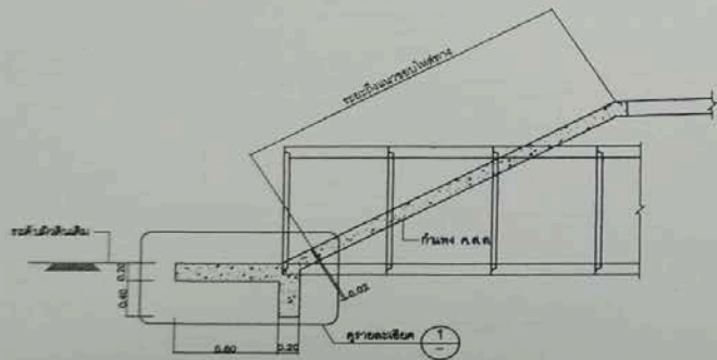
รูปตัดตามยาวแสดงติดตั้ง NOT TO SCALE
