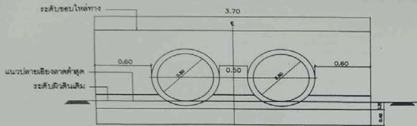
รูปด้านหน้า NOT TO SCALE
