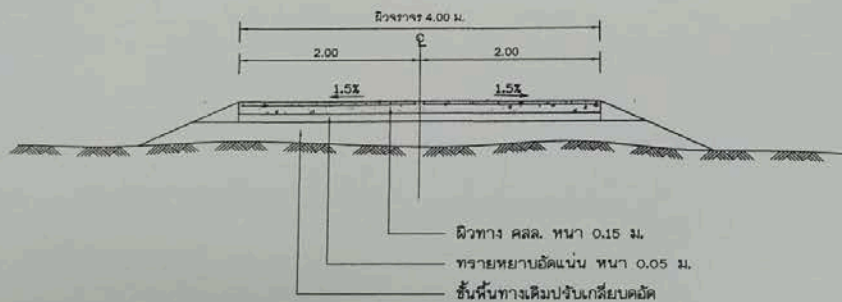
รูปตัดถนน NOT TO SCALE
